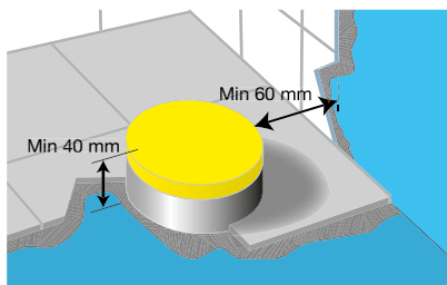
Fig 3.3.1c. Avsättning
