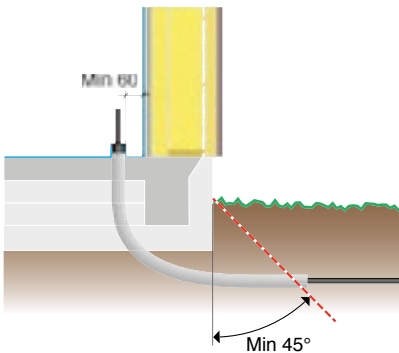
Fig. 3.2.2. Tappvattenservis
